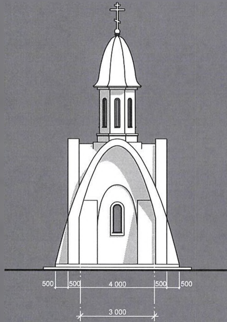
ПІВДЕННИЙ ФАСАД М 1:200
