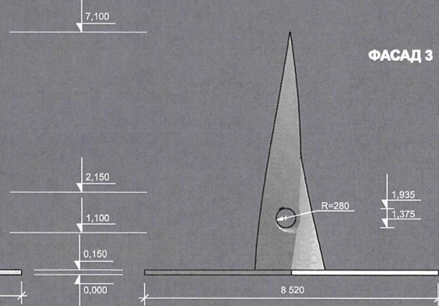
ПАМ'ЯТНА ІМЕННА ПРИЗМА М 1:50
